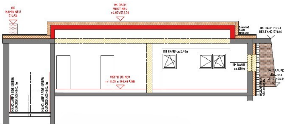
Schnitt C-C
