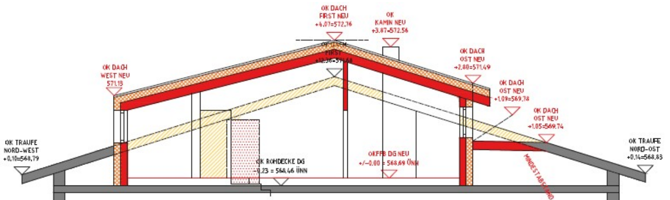
Schnitt B-B
