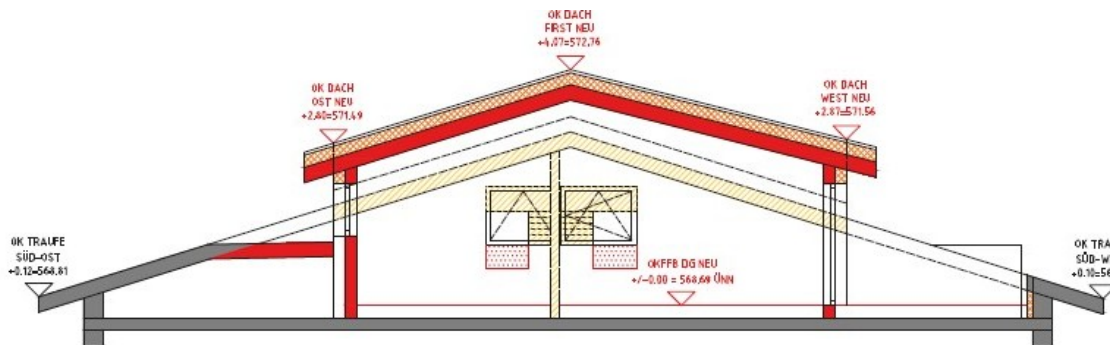
Schnitt B-B
